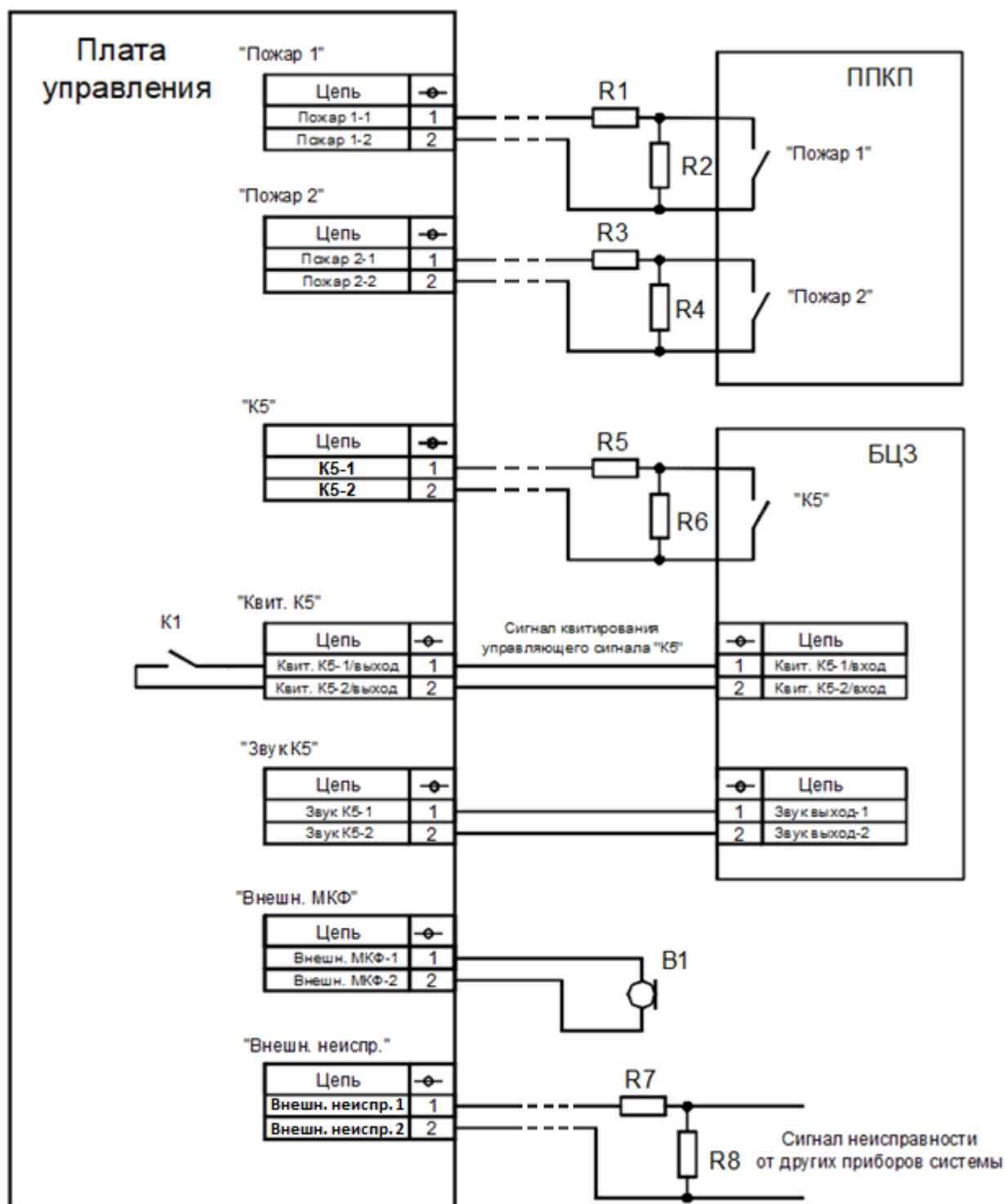
б) Соединение ППУ с ППКП и БЦЗ
